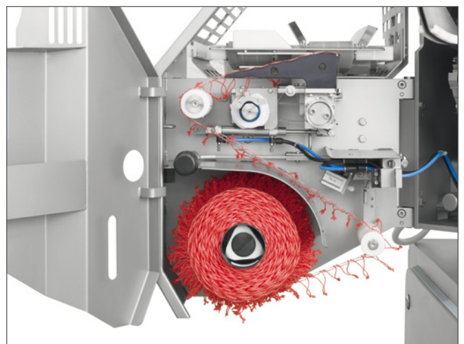
挂绳喂入机构 (BSZ105-2)
