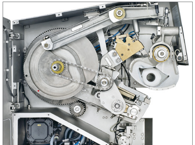
所有驱动摆杆均为一次性不锈钢整体铸造。NewCon® 控制卡扣闭合高度，增加生产可靠性。
