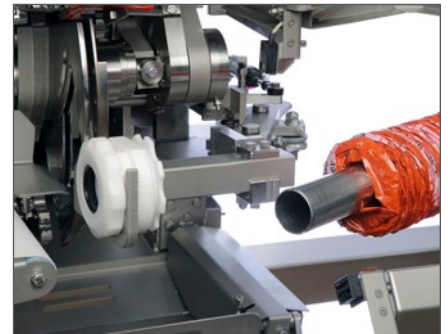
Mecanismo "Quick-Release" para un cambio rápido de la tripa
