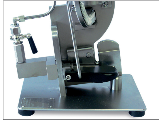
Accionamiento de la palanca de detección y cuchilla desconectable.
