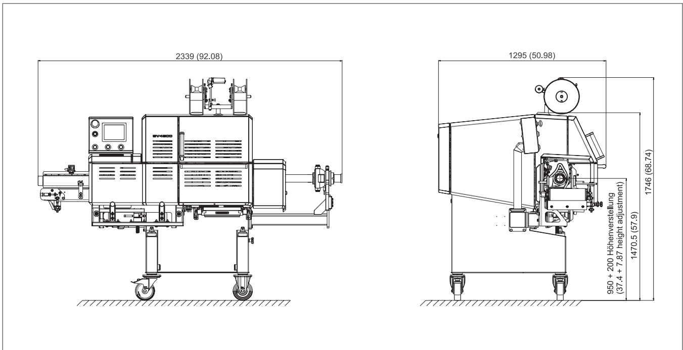
Maße in mm (Zoll)
