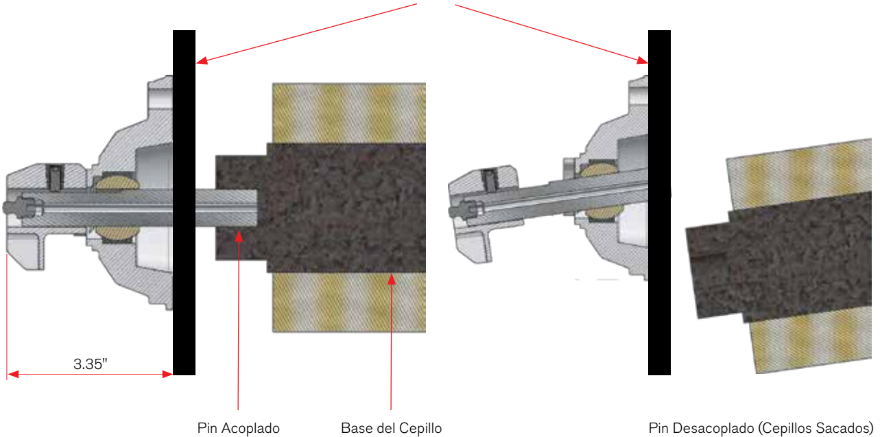
Estructura de la Mesa de Cepillos
